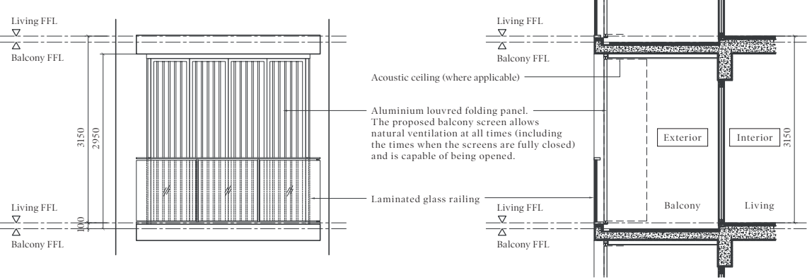
ELEVATION
